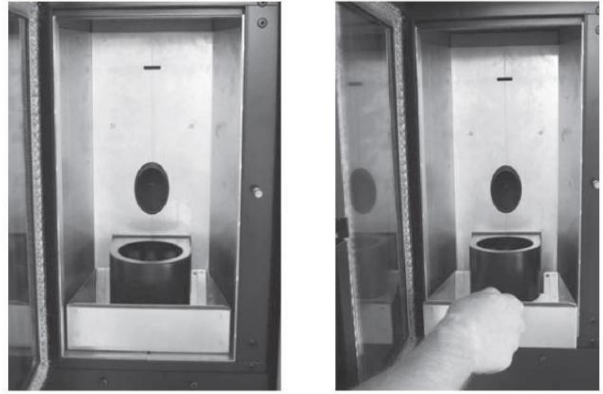
Fig. 18-19: limpieza del contenedor de cenizas
