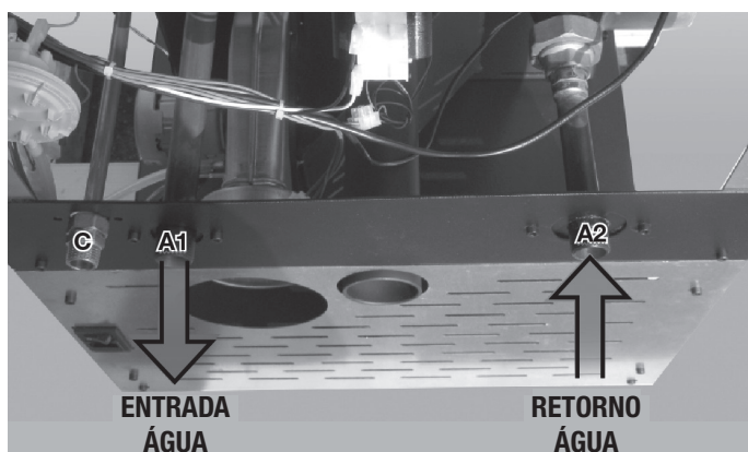
Diagrama de ligação para termo estufa sem kit de água quente sanitária
