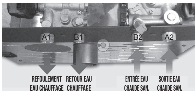
Schéma raccordement hydropoêle avec kit production eau sanitaire
