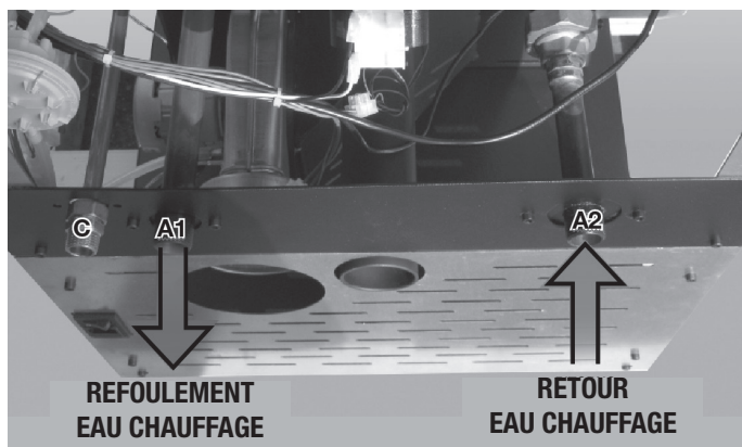
Schéma raccordement hydropoêle sans kit production eau sanitaire
