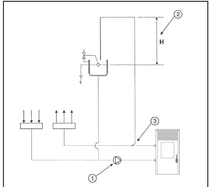
Schema Anschlussleitung Heizofen ohne Brauchwasser-Set
