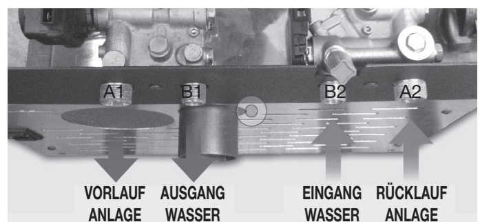
Schema Anschlussleitung Heizofen mit Brauchwasser-Set
