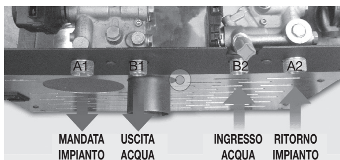
Schema allacciamento termostufa con kit acqua sanitaria
